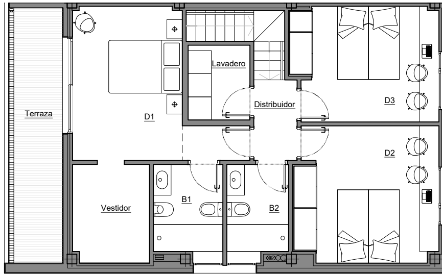
PLANTA PRIMERA
